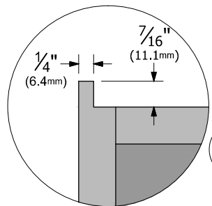
D103 Dovetail Pullout
